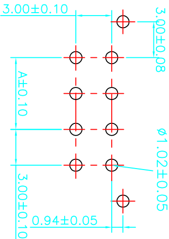
P.C.B LAYOUT
