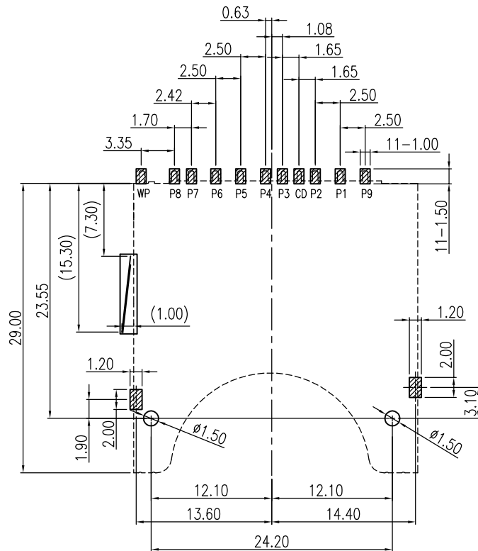
P.C.B LAYOUT
